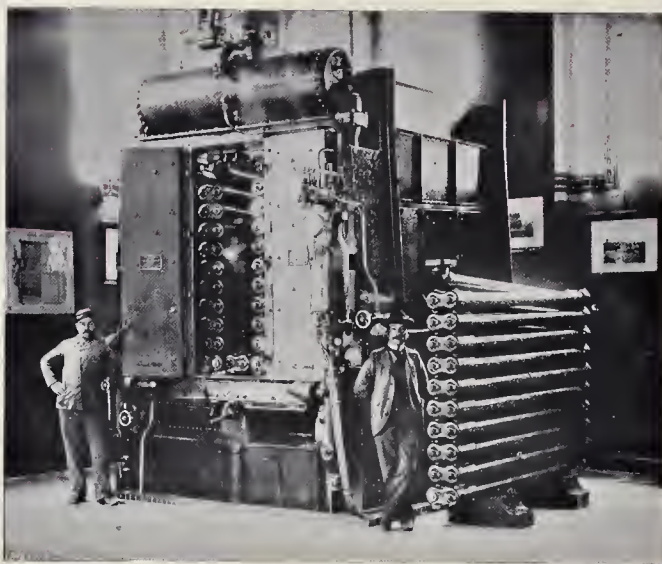
CALDAIA TIPO BELLEVILLE — (PADIGLIONE G. ANSALDO & C.)
